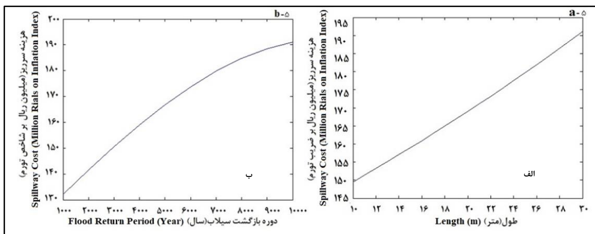
شکل ۵- الف) نمودار هزینه ساخت سرریز و طول آن با فرض T=10000 و هزینه کمینه و ب) نمودار هزینه ساخت سرریز و دوره بازگشت آن با فرض L=10 و هزینه کمینه
