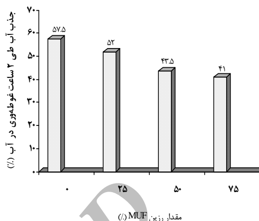
شکل ۶- اثر مستقل نسبت رزین بر جذب آب طی ۲ ساعت
