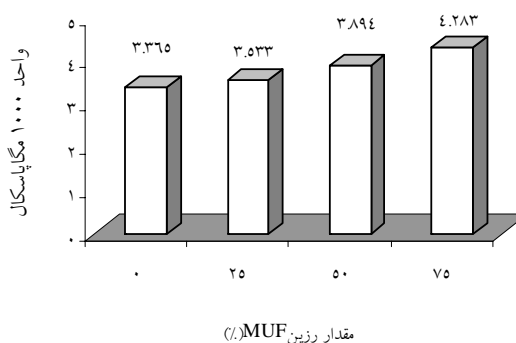
شکل ۲- اثر مستقل نسبت رزین بر مدول الاستیسیته
