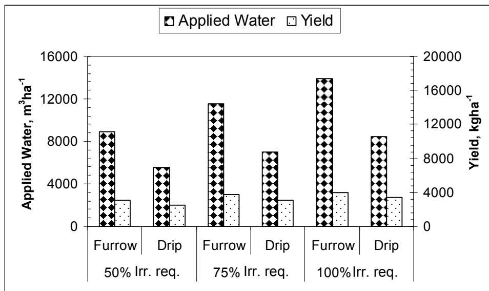
شکل ۲- آب کاربردی و عملکرد و ش در روش آبیاری قطره و شیاری (میانگین دوسال)
