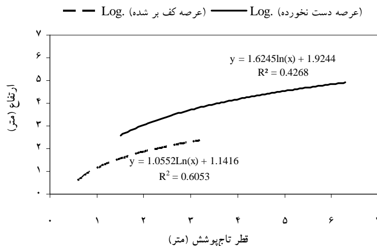
شکل ۴- منحنی ارتفاع توده‌های تاغ در دو عرصه مورد مطالعه
