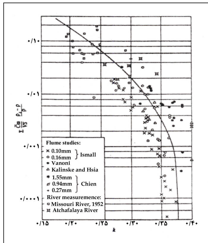
شکل شماره ۱- اثر بار معلق بر پارامتر K ، از: (Einstein & Chien, 1954)
