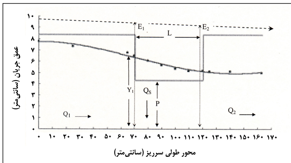
شکل شماره ۷- اجزای سرریز جانبی و تغییرات پروفیل سطح آب در محل سرریز جانبی
