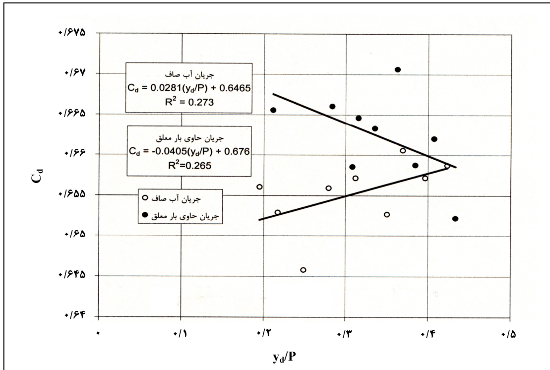
شکل شماره ۳- تأثیر بار معلق جریان بر ضریب شدت جریان سرریز نرمال (Aberi Forutan, 2003)
