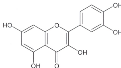
شکل ۲- ساختمان گسترده ترکیب کوئرستین
