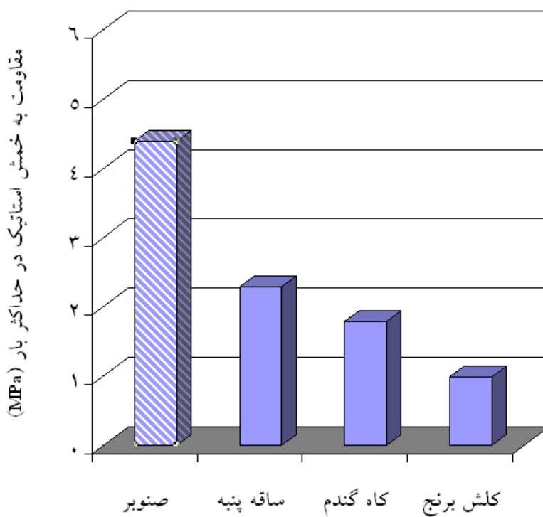
نمودار ۵- مقاومت به خمش استاتیکی در حداکثر بار
