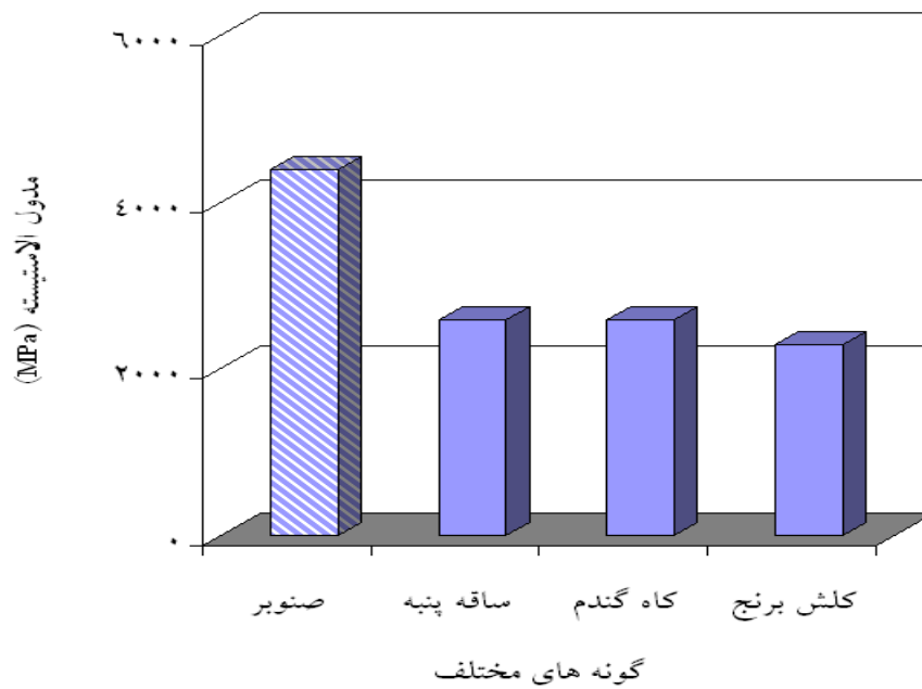
نمودار ۶- مدول الاستیسیته
