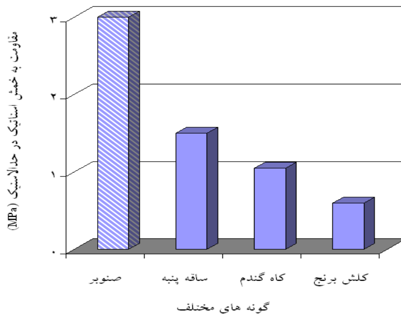
نمودار ۷- مقاومت به خمش در حد الاستیک
