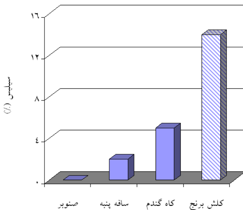
نمودار ۴- تغییرات درصد سیلیس در گونه های مورد آزمایش
