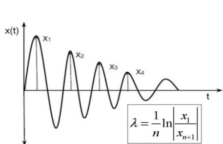
شکل ۱- نمایش فاکتور کاهش: سمت چپ به روش لحظه‌ای با استفاده از کاهش لگاریتمی \lambda ، و سمت راست به روش فرکانسی با استفاده از پهنای باند قله بلندی ارتعاش (فاکتور کیفیت Q)
