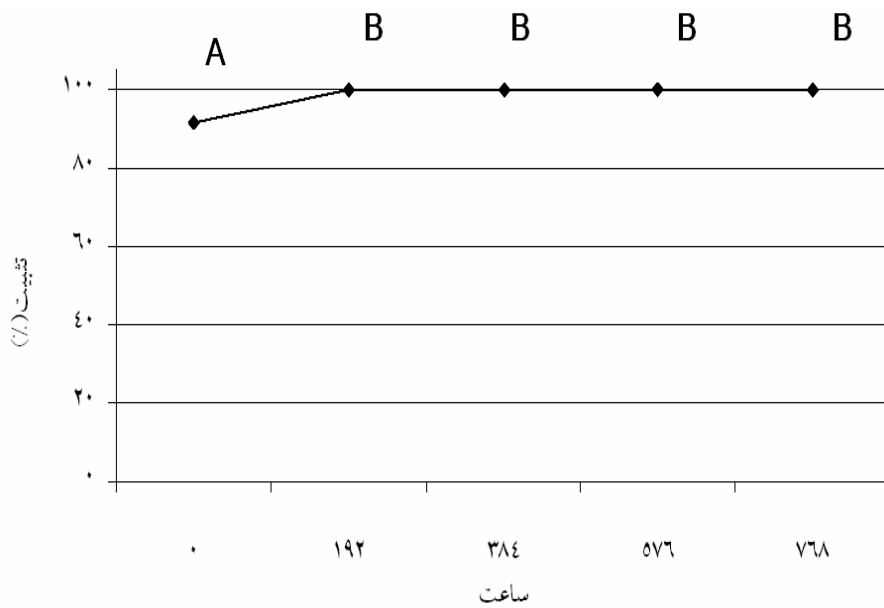
شکل ۶- مقایسه اثر مستقل زمان بر تثبیت کروم (کاهش کروم شش ظرفیتی به کروم سه ظرفیتی) (حروف متشابه مبین عدم تفاوت معنی داری و حروف نامتشابه نشانگر تفاوت معنی داری است ( P > 0.01 )).
