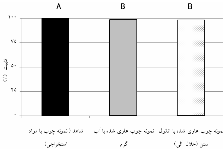
شکل ۳- مقایسه اثر مستقل ماده استخراجی بر مقدار تثبیت کروم (کاهش کروم شش ظرفیتی به سه ظرفیتی) در نمونه‌های چوبی از طریق آزمون چند دامنه‌ای دانکن. حروف مشابه مبین عدم تفاوت معنی‌داری و حروف نامتشابه نشانگر تفاوت معنی‌داری است ( P > 0.01 ).
