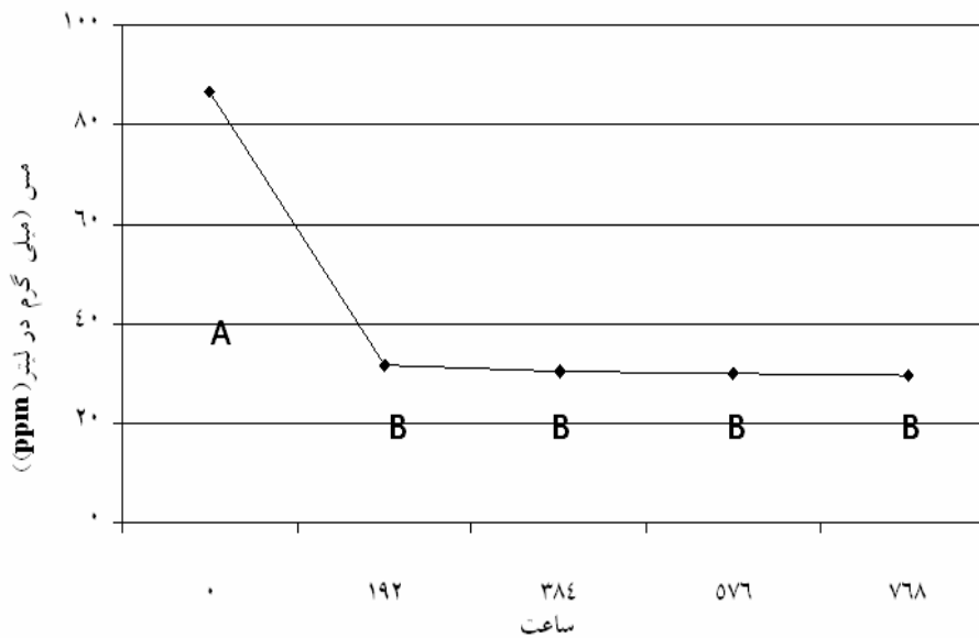
شکل ۴- مقایسه اثر مستقل زمان بر غلظت مس (مس تثبیت نشده) (حروف مشابه مبین عدم تفاوت معنی‌داری و حروف نامتشابه نشانگر تفاوت معنی‌داری است ( P > 0.01 )).
