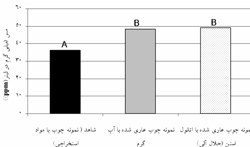
شکل ۲- مقایسه اثر مستقل ماده استخراجی بر غلظت مس موجود در عصاره (مس تثبیت نشده) از طریق آزمون چند دامنه‌ای دانکن (حروف متشابه مبین عدم تفاوت معنی‌داری و حروف نامتشابه نشانگر تفاوت معنی‌داری است) (P>0.01) .
