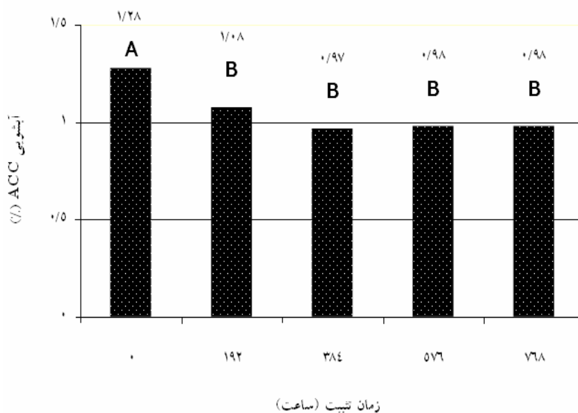
شکل ۸- اثر زمان تثبیت بر آبشویی ماده حفاظتی ACC (حروف متشابه مبین عدم تفاوت معنی داری و حروف نامتشابه نشانگر تفاوت معنی داری بین متوسط داده هاست ( P < 0.01 )).
