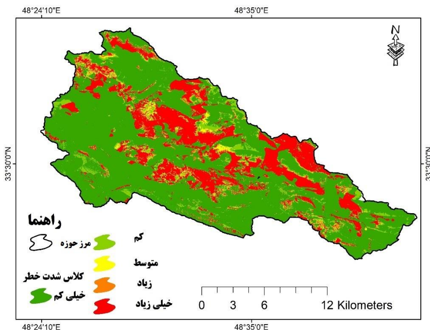
شکل ۳: نقشه شدت حساسیت‌پذیری زمین‌لغزش با مدل جنگل تصادفی در حوزه آبخیز کرگانه
