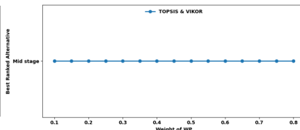
شکل ۴- ارزیابی حساسیت رتبه‌بندی مراحل رشد به تغییرات وزن معیارها
