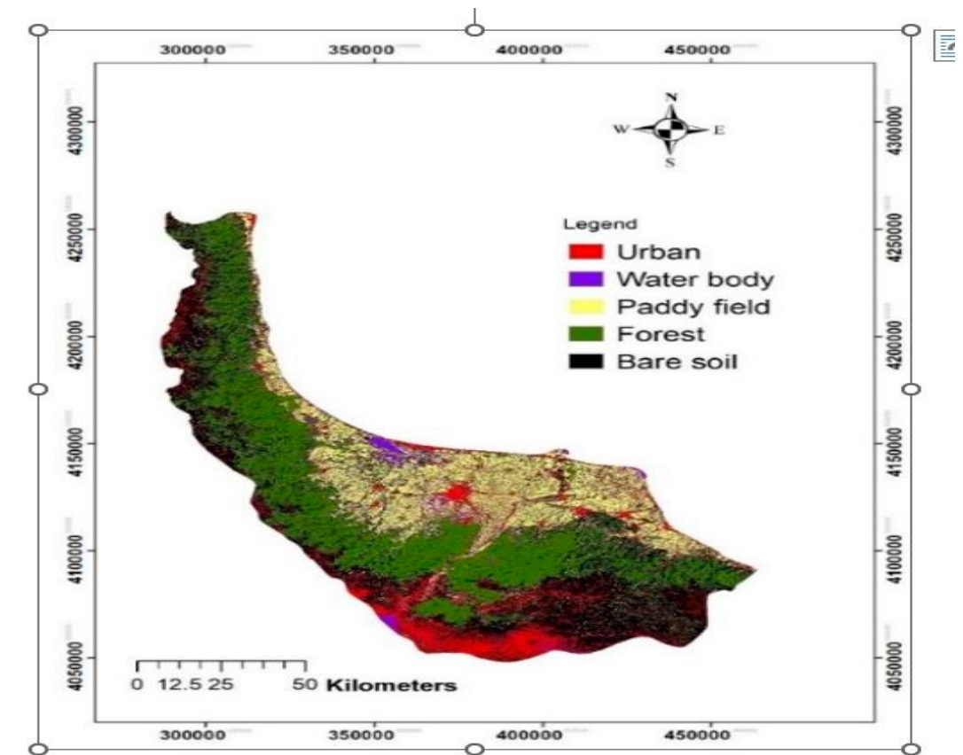
شکل ۱. نقشه کاربری اراضی استان گیلان با استفاده از هوش مصنوعی
