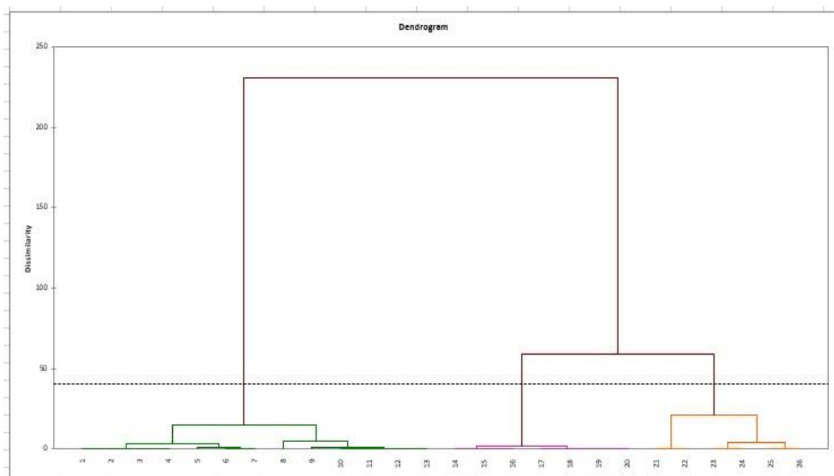
شکل ۱- دندروگرام تجزیه خوشه‌ای ژنوتیپ‌های توتون از نظر صفات مورد مطالعه برای مقاومت به بیماری ساق سیاه در گلخانه
