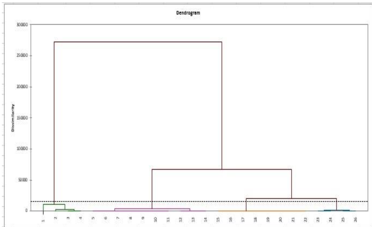
شکل ۲- دندروگرام تجزیه خوشه‌ای ژنوتیپ‌های توتون از نظر صفات مورد مطالعه برای مقاومت به بیماری ساق سیاه در مزرعه Figure 2. Dendrogram of cluster analysis of tobacco genotypes for studied traits to resistance of Black shank disease in field
