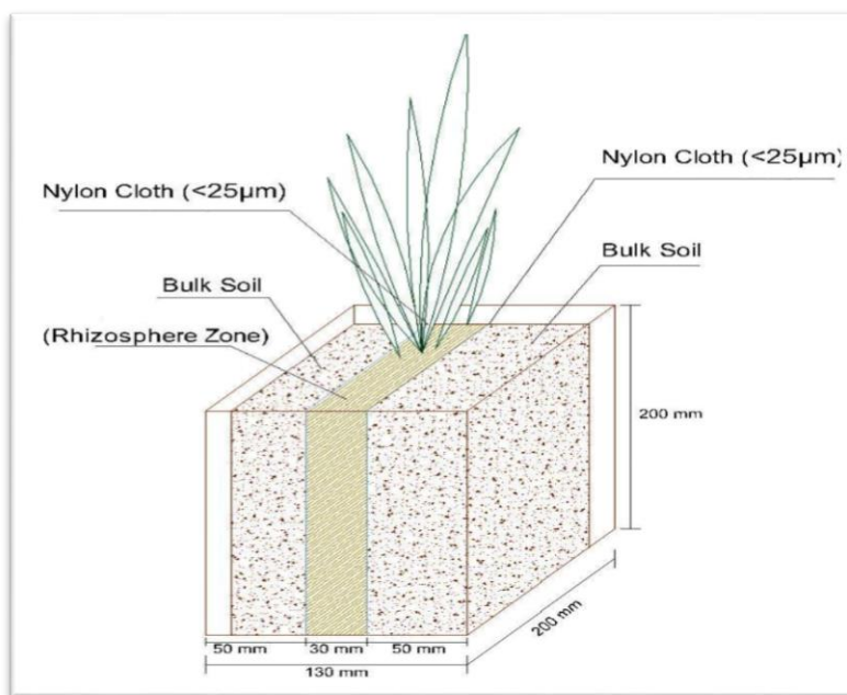
شکل ۱- شماتیک ریزوباکس
