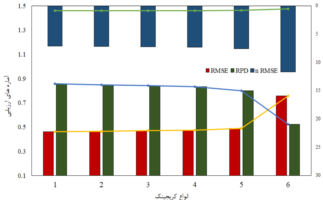
شکل ۵- آماره‌های ارزیابی مربوط به بررسی عملکرد انواع نیم تغییرنما (۱، ۲، ۳، ۴، ۵ و ۶ به ترتیب نمایانگر کریجینگ معمولی با نیم تغییرنماهای کروی، دایره‌ای، نمایی، گوسی، خطی و کریجینگ جهانی یا کریجینگ روند خطی می‌باشند).
