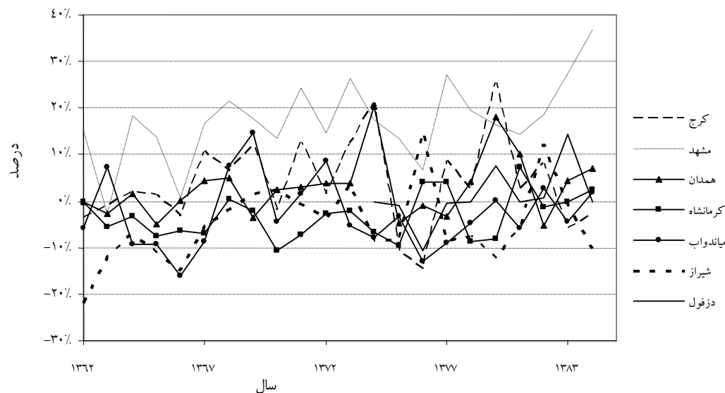
شکل ۱ روند پارامتر جایجایی منحنی عرضه شکر در ایستگاه‌های هفت‌گانه از سال ۱۳۶۲-۱۳۸۳
