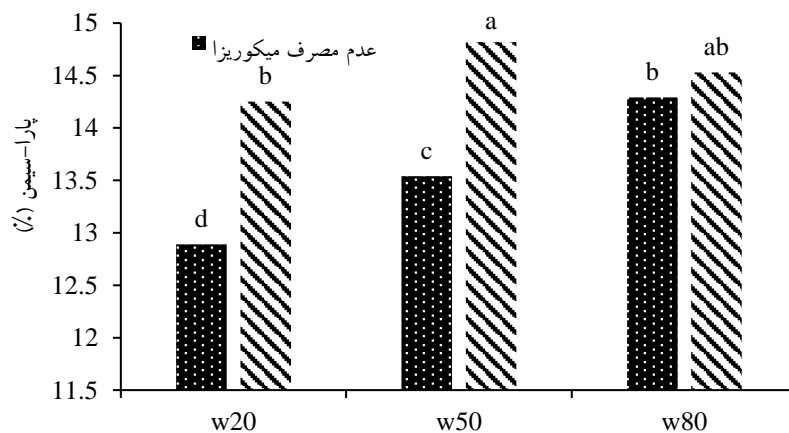
شکل ۵- میزان پارا-سیمن در سطوح مختلف آبیاری با کاربرد قارچ میکوریز
