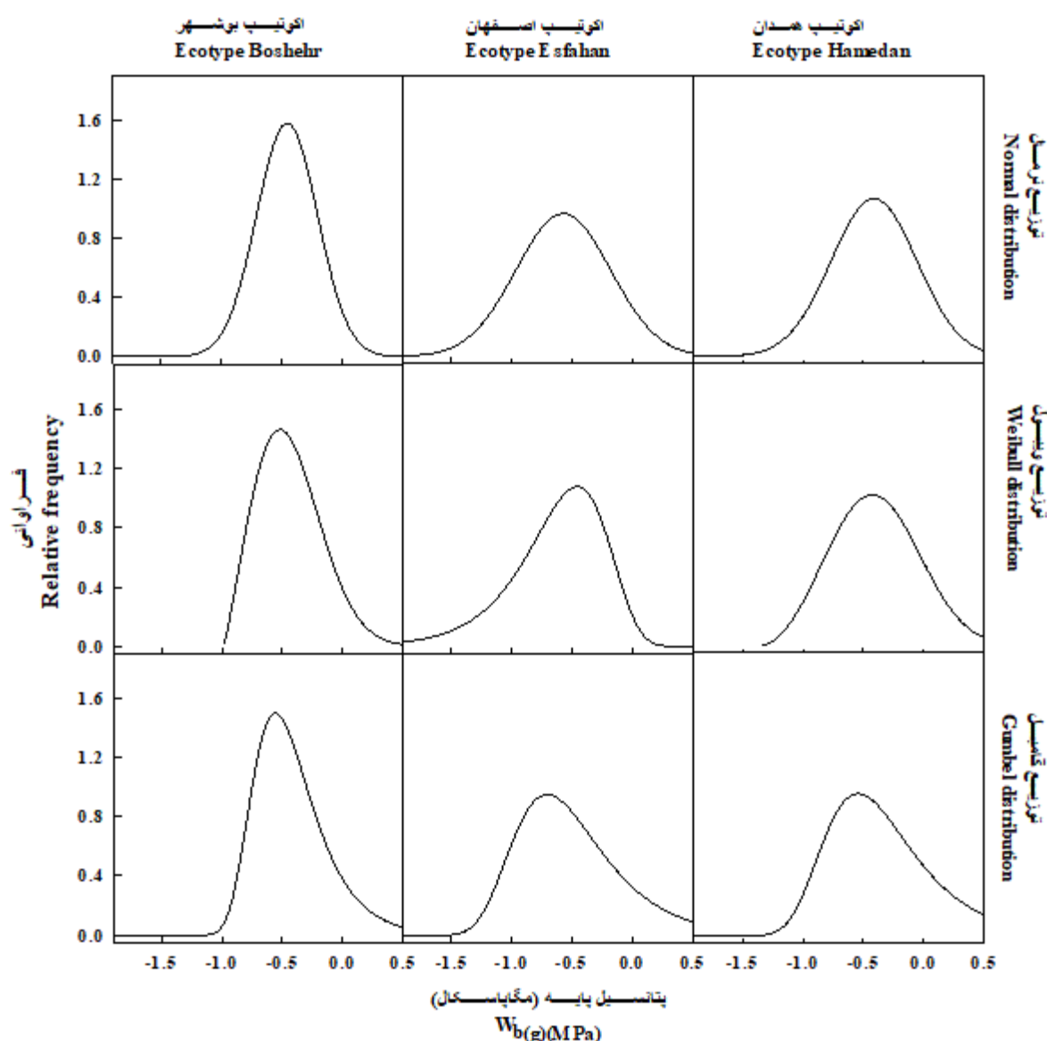
شکل ۳- تابع توزیع احتمال پتانسیل آب پایه پیش بینی شده با مدل هیدروتایم توسعه یافته بر مبنای توزیع های مختلف برای اکوتیپ های مختلف رازیانه. Fig. 3- Probability distribution function of the predicted base water potential for the hydrotime model based on the different distribution for ecotypes fennel.
