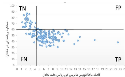
شکل 4- ترسیم گروه‌بندی کیت نلسون برای عملکرد ریشه و فاصله ماهالانویس - هفت تعادل
