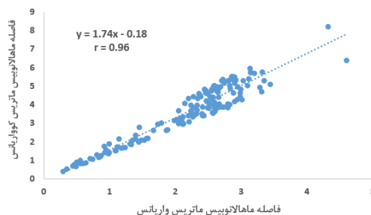
شکل 10- ارتباط بین فاصله مآهالاتوبیس کواریانس ماتریس (ilr) و فاصله مآهالاتوبیس ماتریس واریانس (ilr) - سه تعادل
