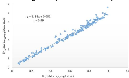
شکل 6- ارتباط بین فاصله ایچسن (ilr) و فاصله مآهالاتوبیس (ilr) - سه تعادل
