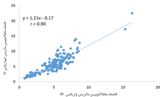
شکل 11- ارتباط بین فاصله مآهالاتوبیس کواریانس ماتریس (ilr) و فاصله مآهالاتوبیس ماتریس واریانس (ilr) - هفت تعادل
