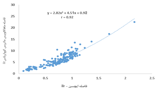
شکل 7- ارتباط بین فاصله ایچسن (ilr) و فاصله مآهالاتوبیس (ilr) - هفت تعادل
