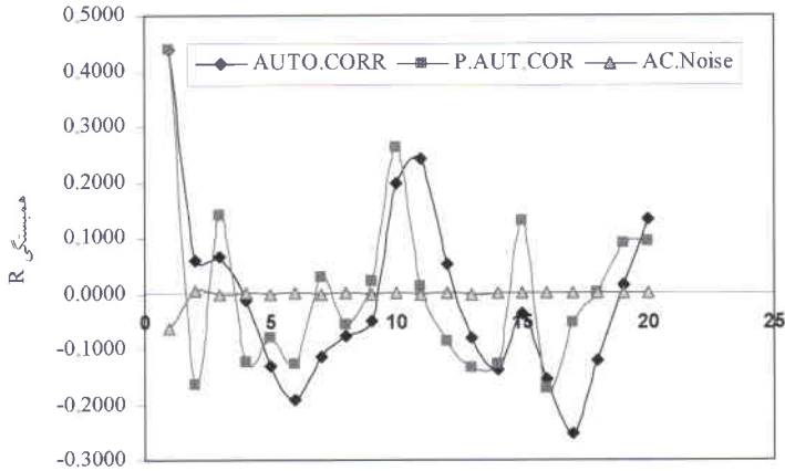
نمودار شماره ۵- تغییرات ضرایب خود همبستگی برای داده‌های ضریب رواناب سالانه در هم‌دوره ۳۰ ساله ۴۶-۱۳۴۵ تا پایان ۷۵-۱۳۷۴ (۲۰ گام ده ساله).
