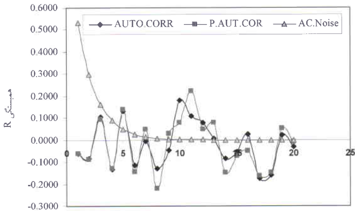
نمودار شماره ۶- تغییرات ضرایب خود همبستگی برای داده‌های ضریب رواناب بهاره در هم‌دوره ۳۰ ساله ۴۶-۱۳۴۵ تا پایان ۷۵-۱۳۷۴ (۲۰ گام ده ساله).
