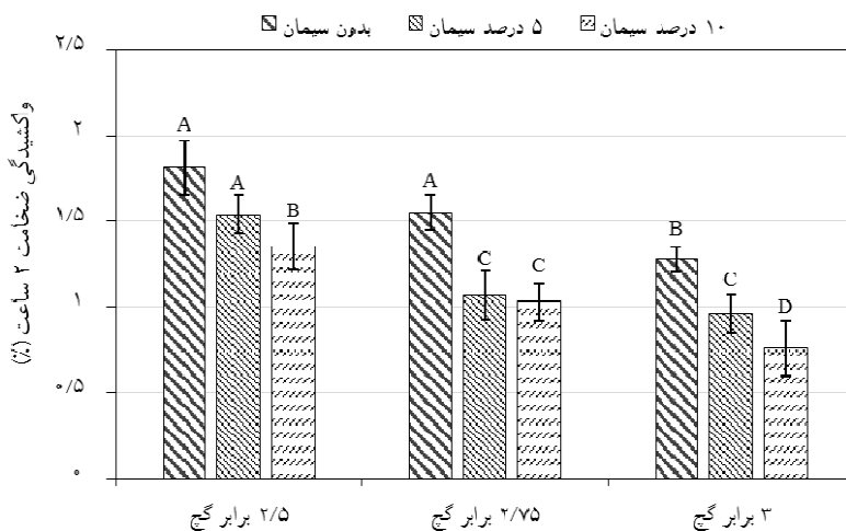
شکل ۳- واكشیدگی ضخامت چوب گچ بعد از ۲ ساعت غوطه‌وری در آب
