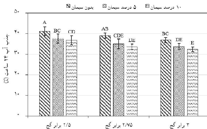
شکل ۲- جذب آب تخته‌های چوب گچ بعد از ۲۴ ساعت غوطه‌وری در آب
