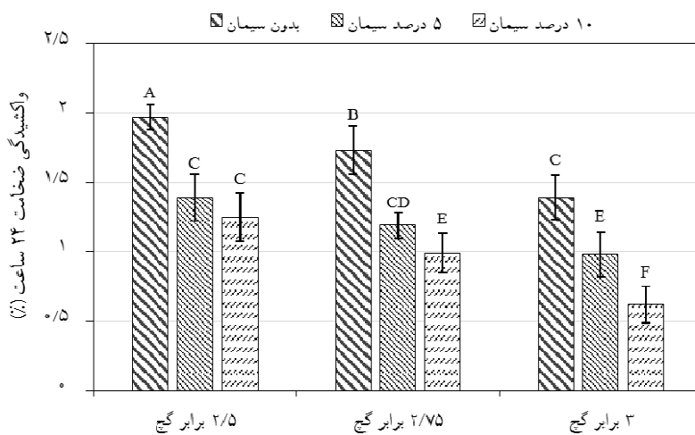
شکل ۴- واكشیدگی ضخامت تخته‌های چوب گچ بعد از ۲۴ ساعت غوطه‌وری در آب
