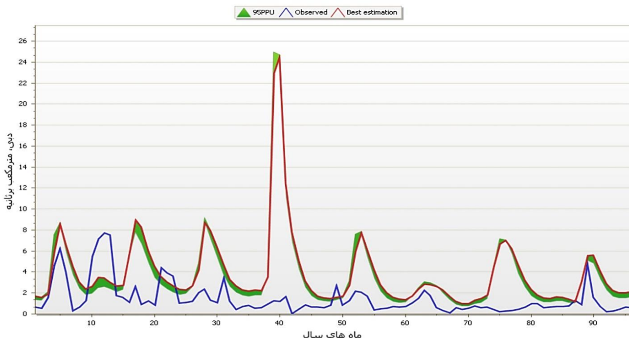
شکل ۷- مقایسه‌ی آب‌دهی‌های مشاهداتی با مقادیر شبیه‌سازی‌شده در مرحله‌ی اعتبارسنجی.
