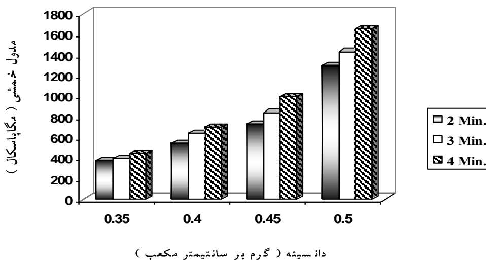
شکل ۴ - اثر متقابل میان دانسیته و زمان پرس بر مدول خمشی تخته خرده چوب عایقی
