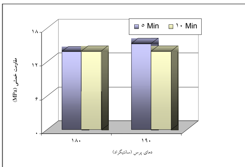
شکل ۱- اثر متقابل زمان بخارزنی و دمای پرس بر مقاومت خمشی
