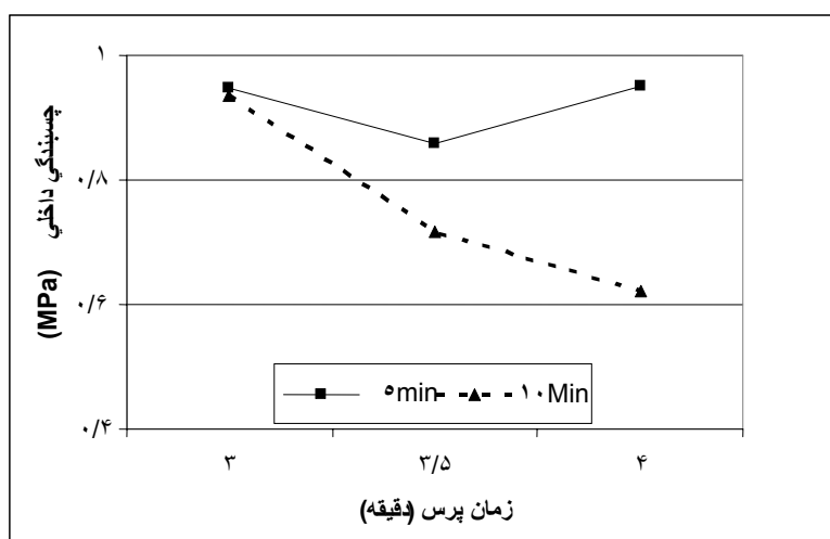
شکل ۴ - اثر متقابل زمان بخارزنی و زمان پرس بر چسبندگی داخلی
