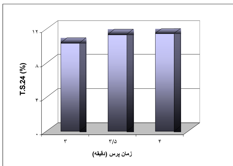
شکل ۵ - اثر زمان پرس بر واکشیدگی ضخامت ۲۴ ساعت
