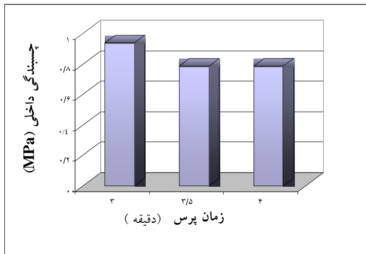
شکل ۳ - اثر زمان پرس بر چسبندگی داخلی
