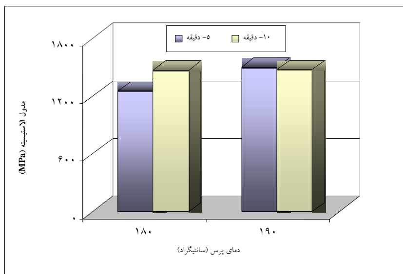
شکل ۲ - اثر متقابل زمان بخارزنی و دمای پرس بر مدول الاستیسیته
