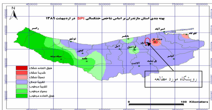
شکل ۱- پهنه‌بندی استان مازندران براساس شاخص خشکسالی SPI در اردیبهشت ۱۳۸۹ و
