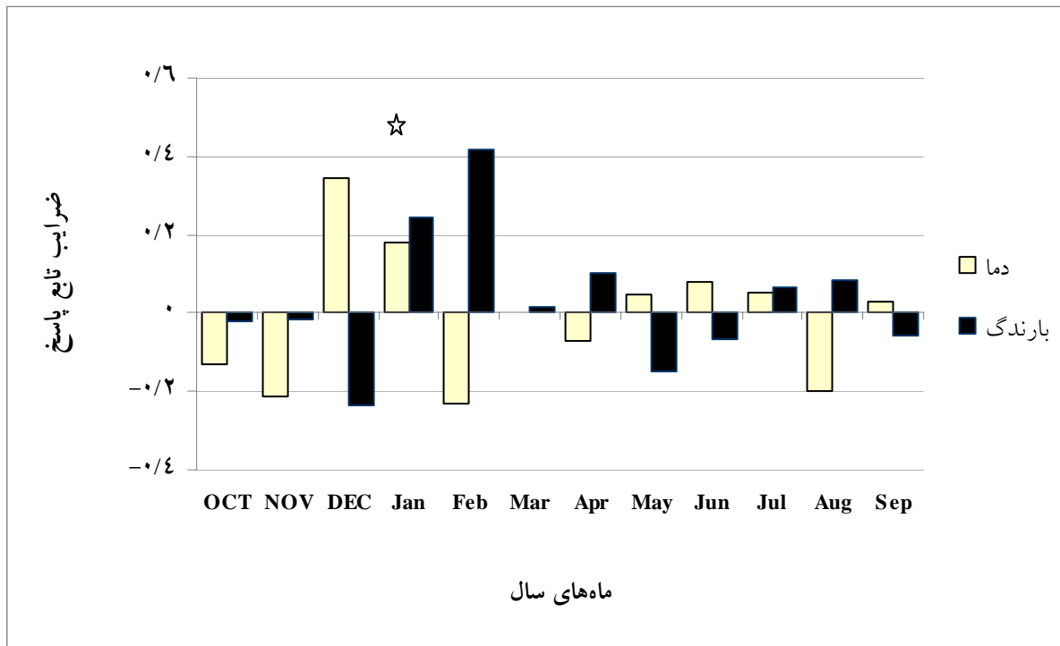
شکل ۵- ضرایب تابع پسخ و شاخص کرونولوژی باقیمانده درخت آزاد (علامت ☆ ماه‌های غنی‌داری را نشان می‌دهد).
