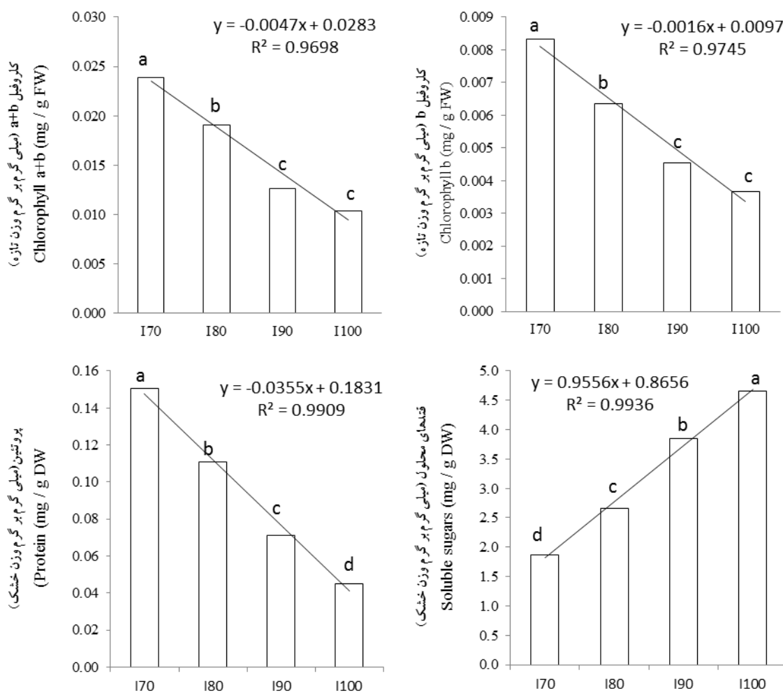
شکل ۲- اثر تنش خشکی بر صفات فیزیولوژیکی در برگ ماش. I70، I80، I90 و I100 تنش خشکی به ترتیب شامل آبیاری پس از ۷۰ (آبیاری نرمال)، ۸۰، ۹۰ و ۱۰۰ میلی متر تبخیر از تشتک تبخیر کلاس الف؛ A0، A50 و A100 به ترتیب عدم کاربرد ریزگرد و کاربرد ۵۰ و ۱۰۰ میلی گرم در متر مکعب ریزگرد.
