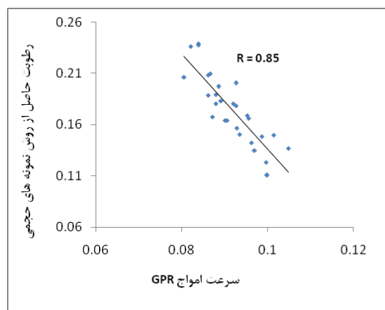
شکل ۹- رابطه‌ی بین سرعت امواج GPR و رطوبت اندازه‌گیری شده با روش حجمی
