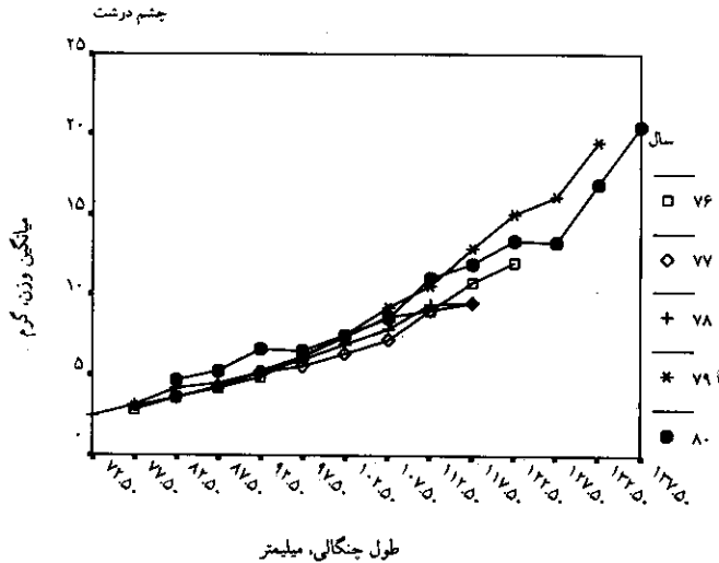
نمودار ۷: میانگین وزن در کلاسهای مختلف طول (چنگالی) کیلکای چشم درشت در سواحل ایران در سالهای ۱۳۷۶ تا ۱۳۸۰
