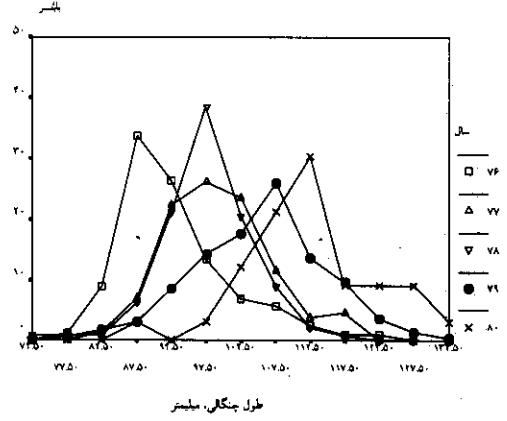
نمودار ۳: فراوانی طول چنگالی کیلکای چشم درشت در منطقه بابل
