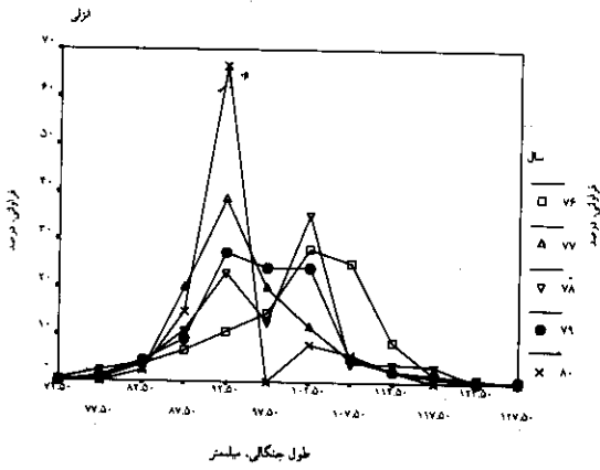
نمودار ۴: فراوانی طول چنگالی کیلکای چشم درشت در منطقه انزلی
