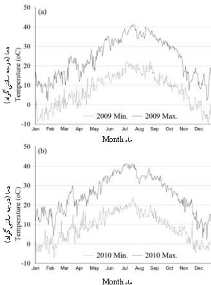
شکل ۱- تغییرات حداقل و حداکثر دمای روزانه در (a) سال ۸۷-۸۸ و (b) سال ۸۸-۸۹ در منطقه مغان Fig. 1. Variation in daily minimum and maximum temperatures (a) 2009 and (b) 2010 in Moghan region
