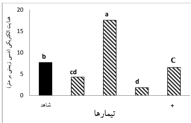
شکل ۲- هدایت الکتریکی خاک در عمق ۰-۳۰ سانتی متر
