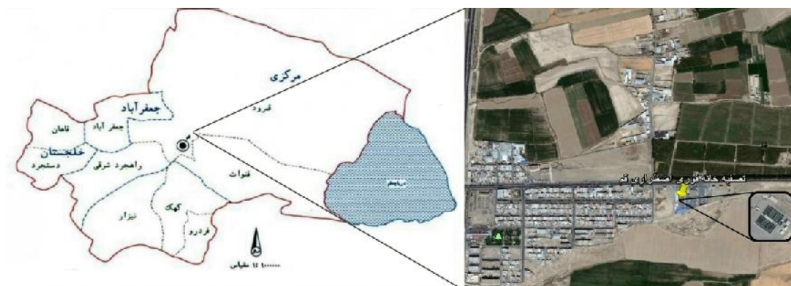
شکل ۱- موقعیت محدوده مطالعه در استان قم
